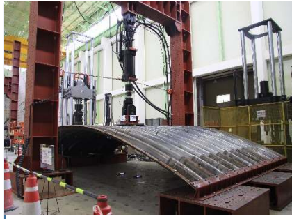
파형강판 방호 성능시험
