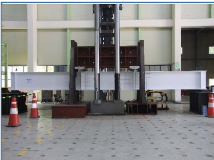
H형강 구조성능 평가시험
